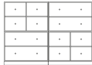
Dresser on plinth W 139.2 cm H 93.6 cm Plinth H 7 cm
